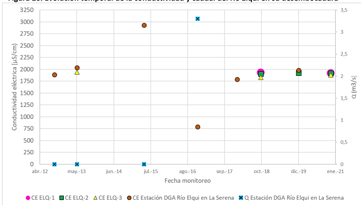
Figura 26. Evolución temporal de la conductividad y caudal del río Elqui en su desembocadura
