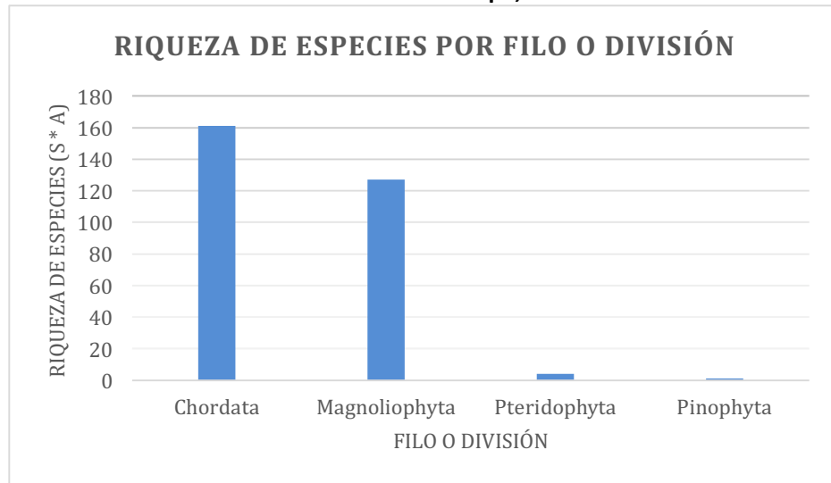
Gráfico 1. Riqueza de especies estandarizada de los filos o divisiones presentes en el humedal de la desembocadura del Elqui, La Serena
