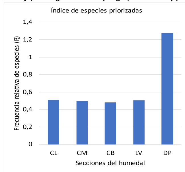
Gráfico 8. Frecuencia relativa de especies priorizadas (endémicas, migratorias y prioritarias) en cada sección del humedal del Elqui, La Serena (CL= curso alto y lagunas, CM= curso medio, CB= curso bajo, LV= laguna costera y vegas, DP= dunas y playa)
