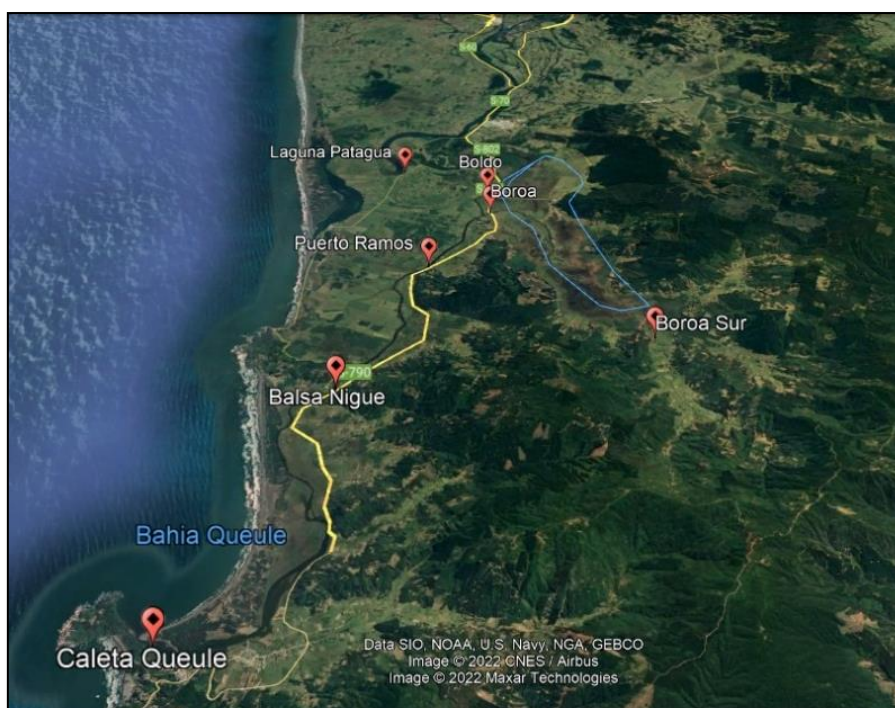
Figura 1. Puntos de muestreo para Macroinvertebrados bentónicos en los humedales del río Queule.
